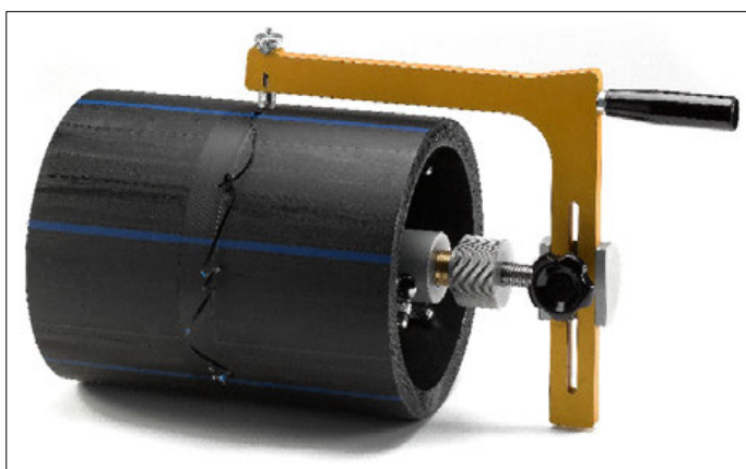
Рис.11. Механический скребок
