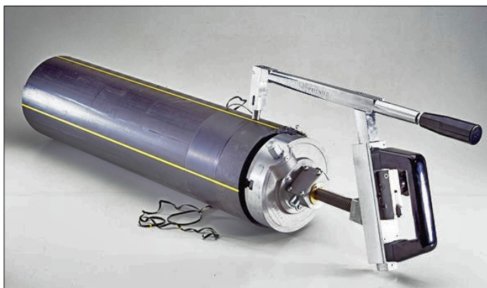
Рис.10. Механический скребок
