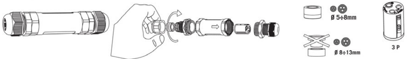
Рис. 32. Разобрать соединительный комплект TH400 3P полностью.
