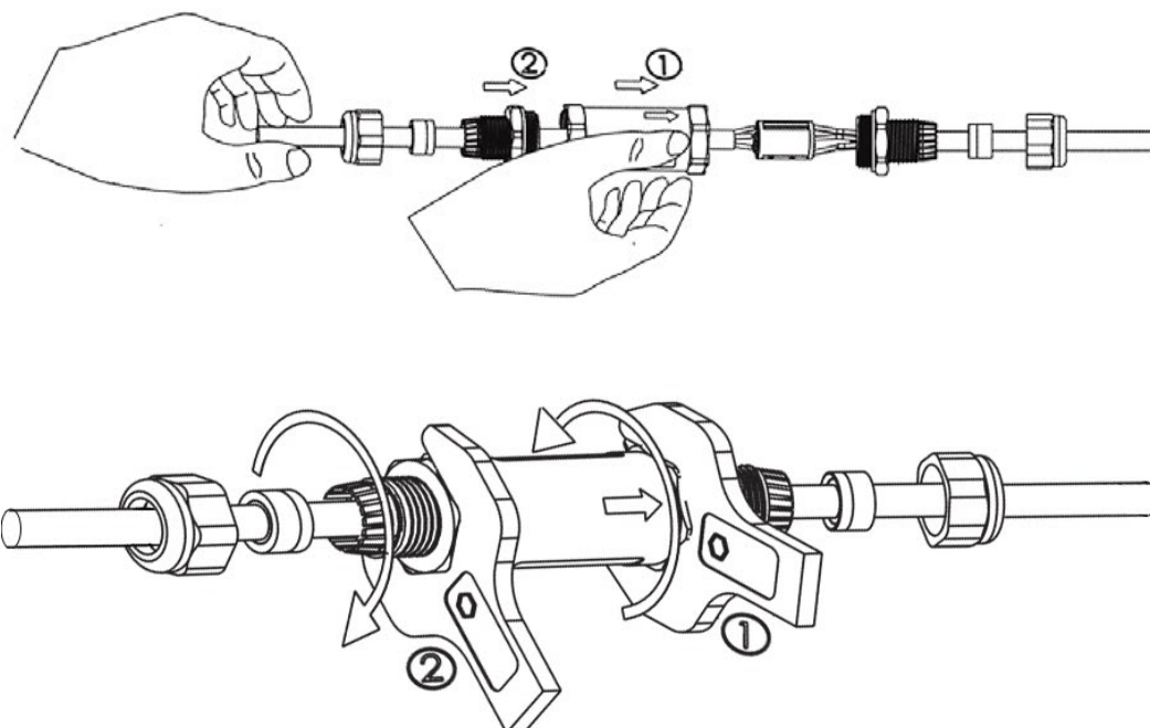
Рис.35. Закрутить обе части
