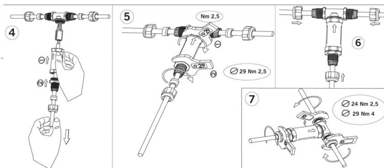
Рис. 36. Последовательность установки кабеля
