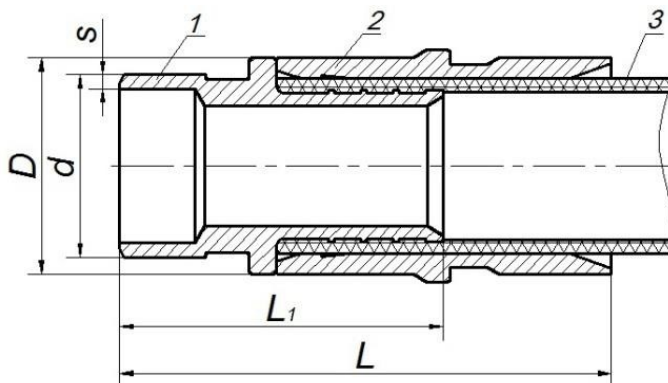
Рис. 5. Монтажная гильза для систем ТВЭЛ-ПЭКС, ТВЭЛ-ПЭКС-К
