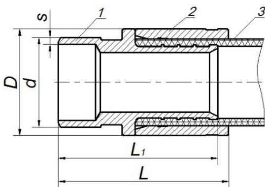
Рис. 6. Переход на сварное соединение с монтажной гильзой для труб ТВЭЛ-ПЭКС
