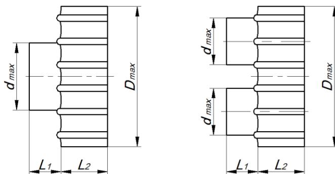
Рис. 18. Термоусаживающаяся заглушка
